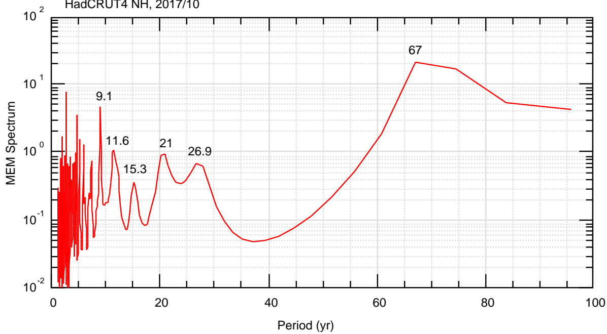
HadCRUT4 NH, 2017/10
