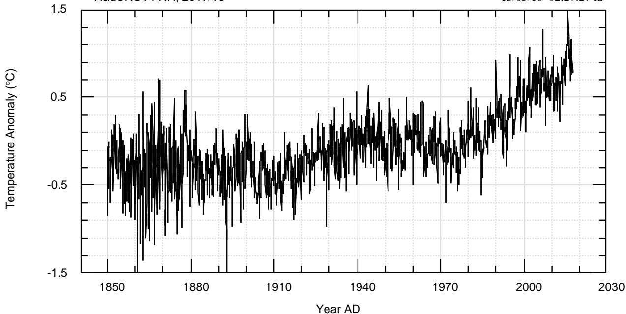
HadCRUT4 NH, 2017/10
