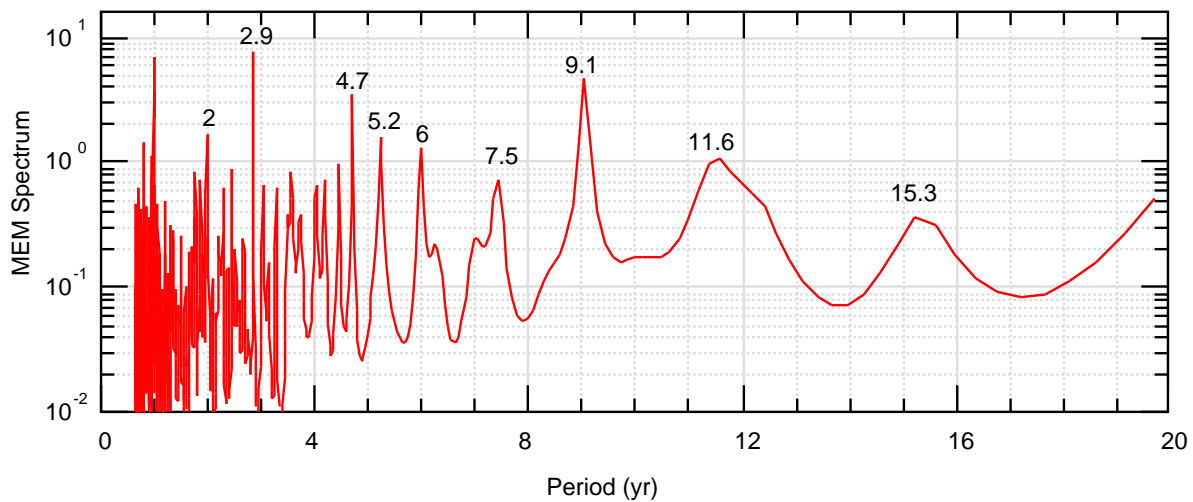
HadCRUT4 NH, 2017/10
