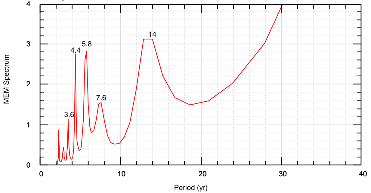
SIV-yr Obs
