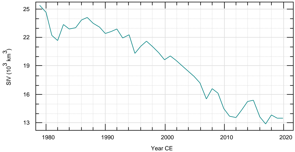
SIV-yr Obs
