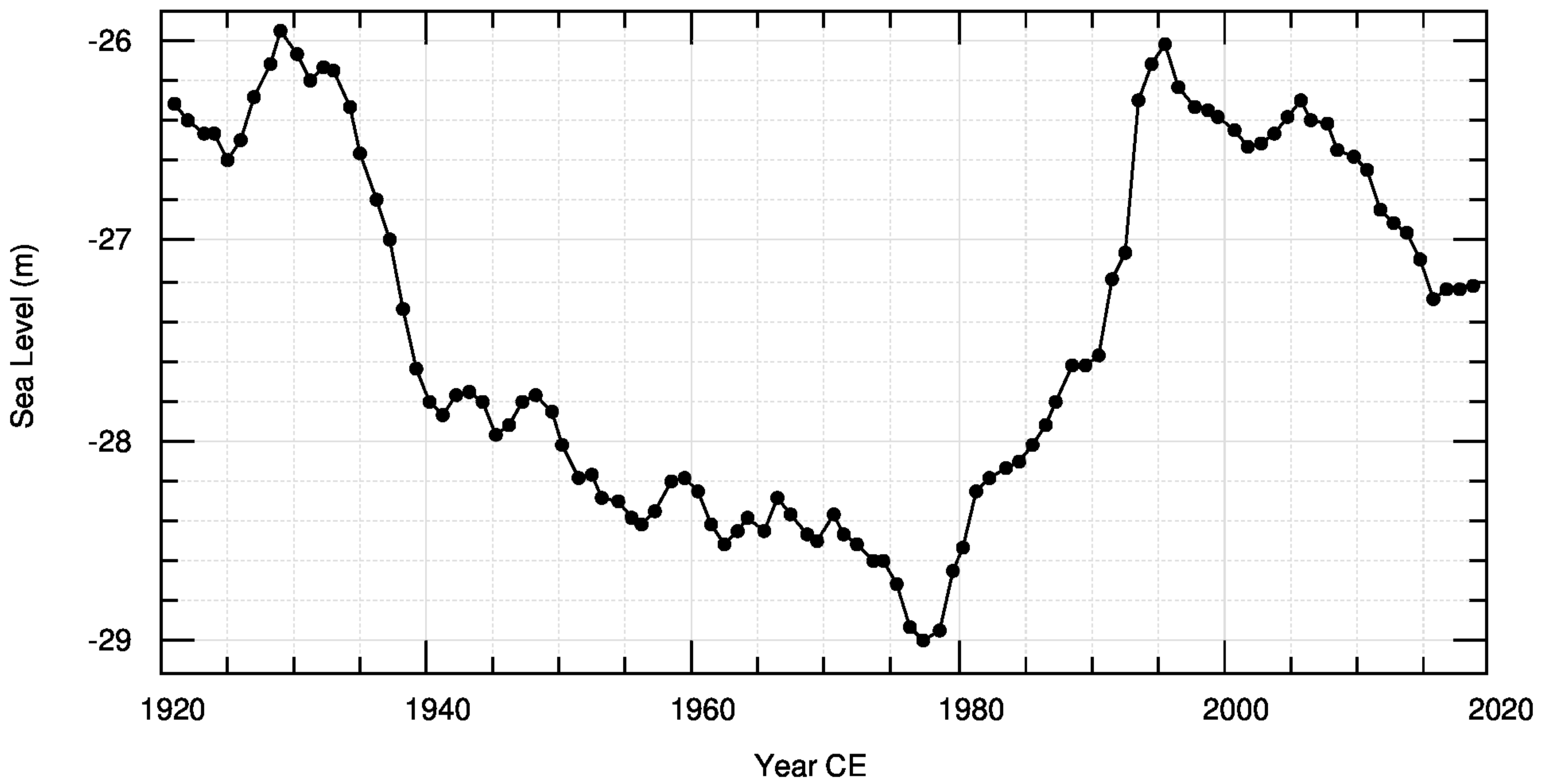
Caspian Sea 1921-2018
