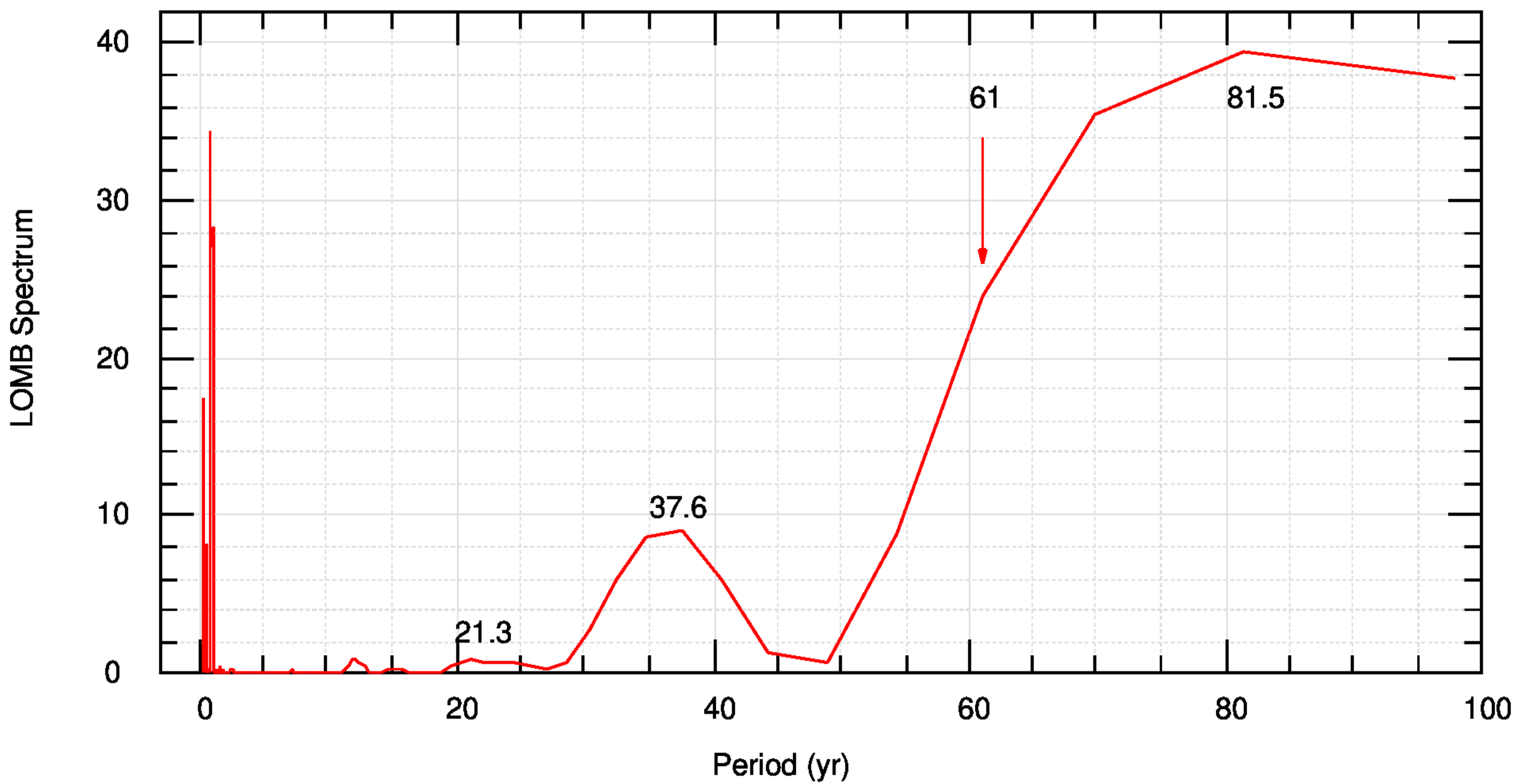
Caspian Sea 1921-2018
