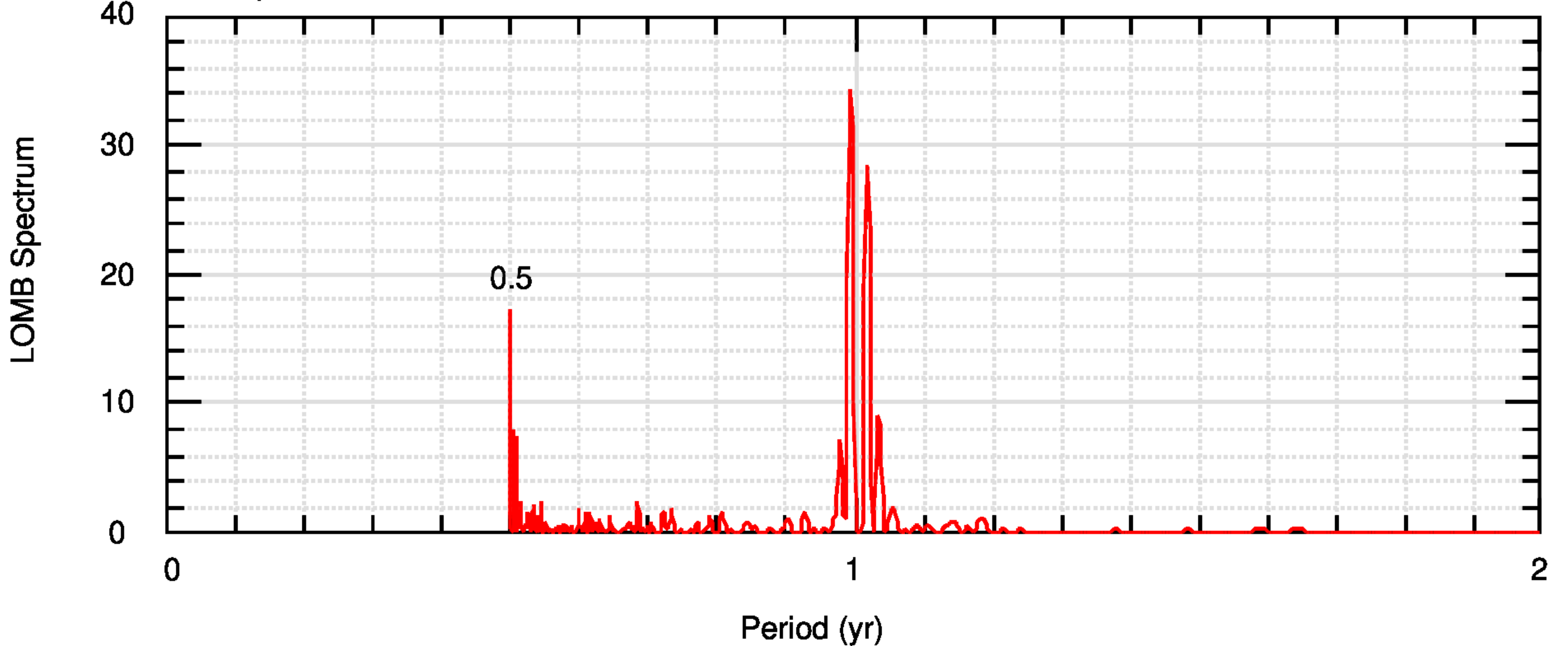
Caspian Sea 1921-2018
